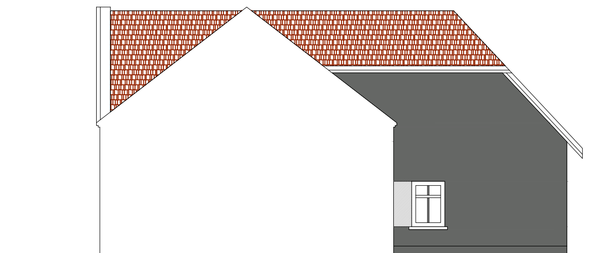
WIDOK 3-3
